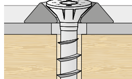
Trou cylindrique avec rondelle fraisée HUS.
