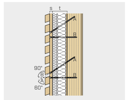
파사드 단열
