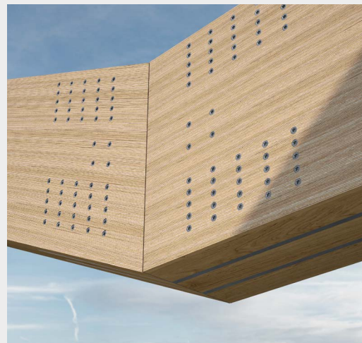
Жесткое угловое соединение с двумя закладными пластинами (ЛВЛ).
