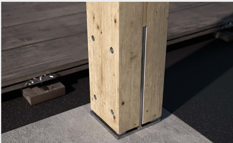
Крепление опоры для колонн Rothoblaas с закладной врезной пластиной F70.
