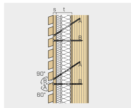
ΜΟΝΩΤΙΚΟ ΠΡΟΣΟΨΗΣ
