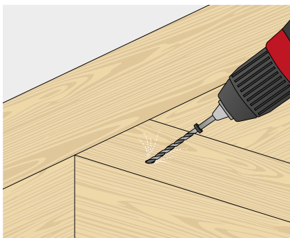
οπή-οδηγός
