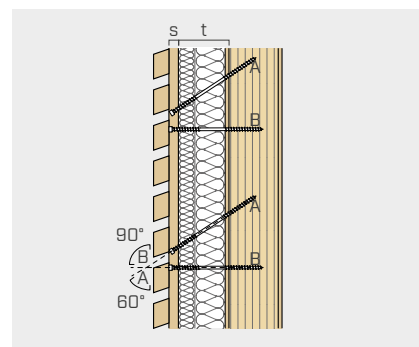
FASÁDNA ISOLÁCIA
