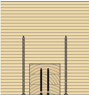
主视图
