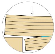
锥形梁 垂直纹理方向的拉力加固
