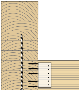
截面图
