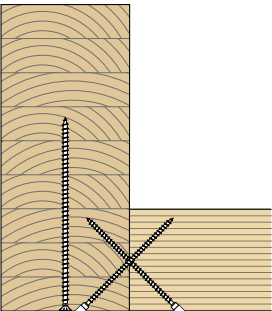
截面图
