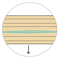
锥形梁 垂直纹理方向的顶点拉力加固
