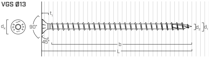
VGS Ø13
