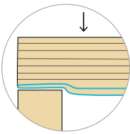
支撑 垂直纹理方向的压力加固
