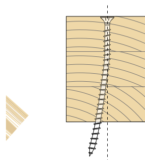
不带预钻孔 的攻入
