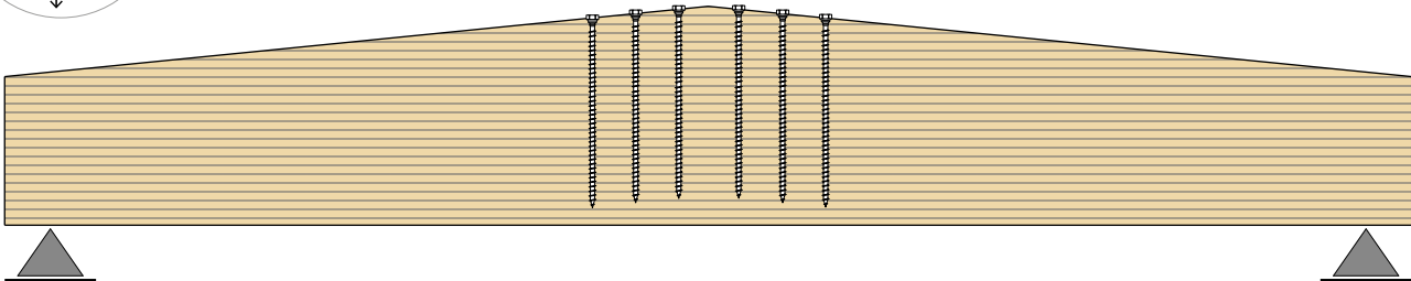
锥形梁 垂直纹理方向的顶点拉力加固
