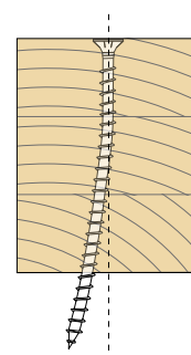
insertion sans trou pilote
