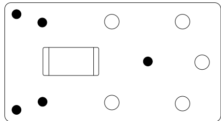
5x agujeros avellanados Ø11 mm
