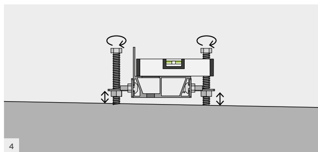
Boční zarovnání profilů.
