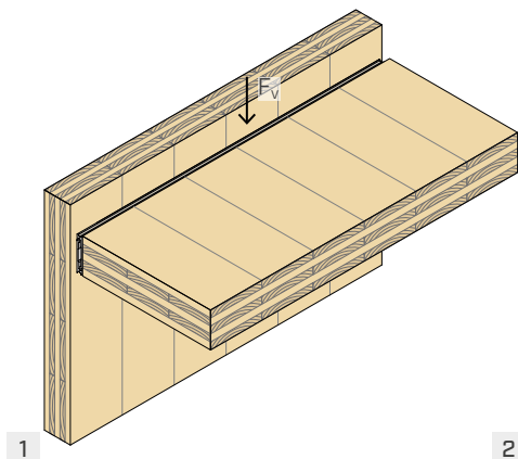
CLT stěna | CLT podlaha
