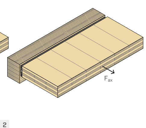
nosník | podlaha CLT
