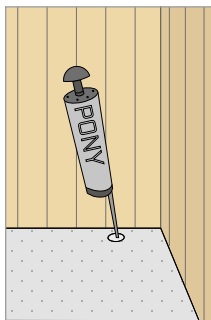
Luknjanje betona in čiščenje izvrtine
