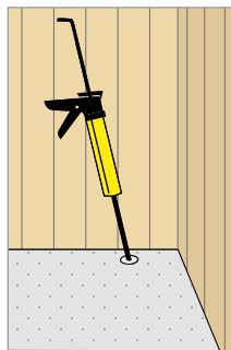
Vbrizganje kemijskega sidrala v luknjo
