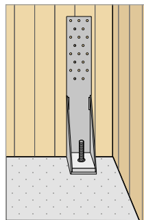
Vgradnja kotnika WHT (s pripadajočo podložko, če je predvidena)
