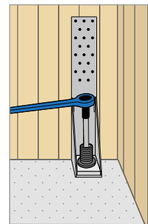
Vstavev matice z ustreznim navojnim privitja
